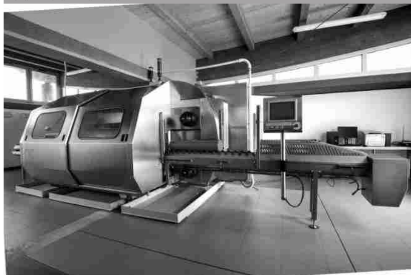
Il pastorizzatore di Villa Food
